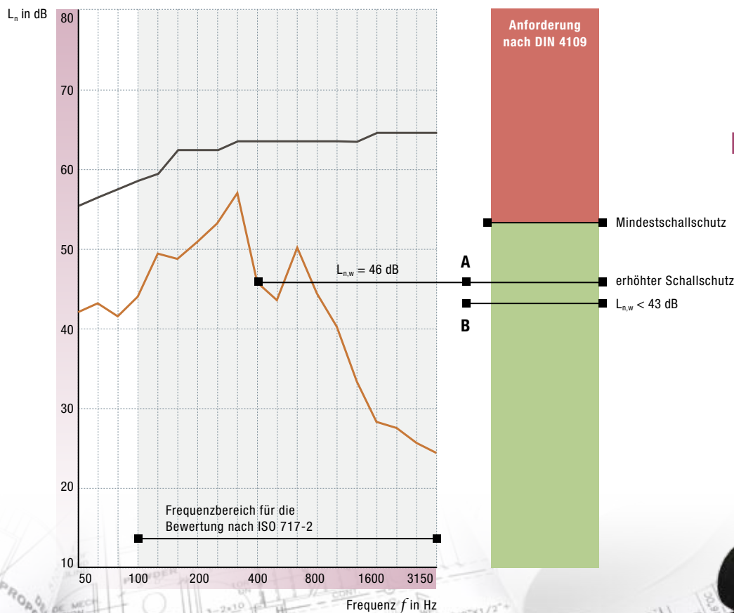
Baustellenmessung
