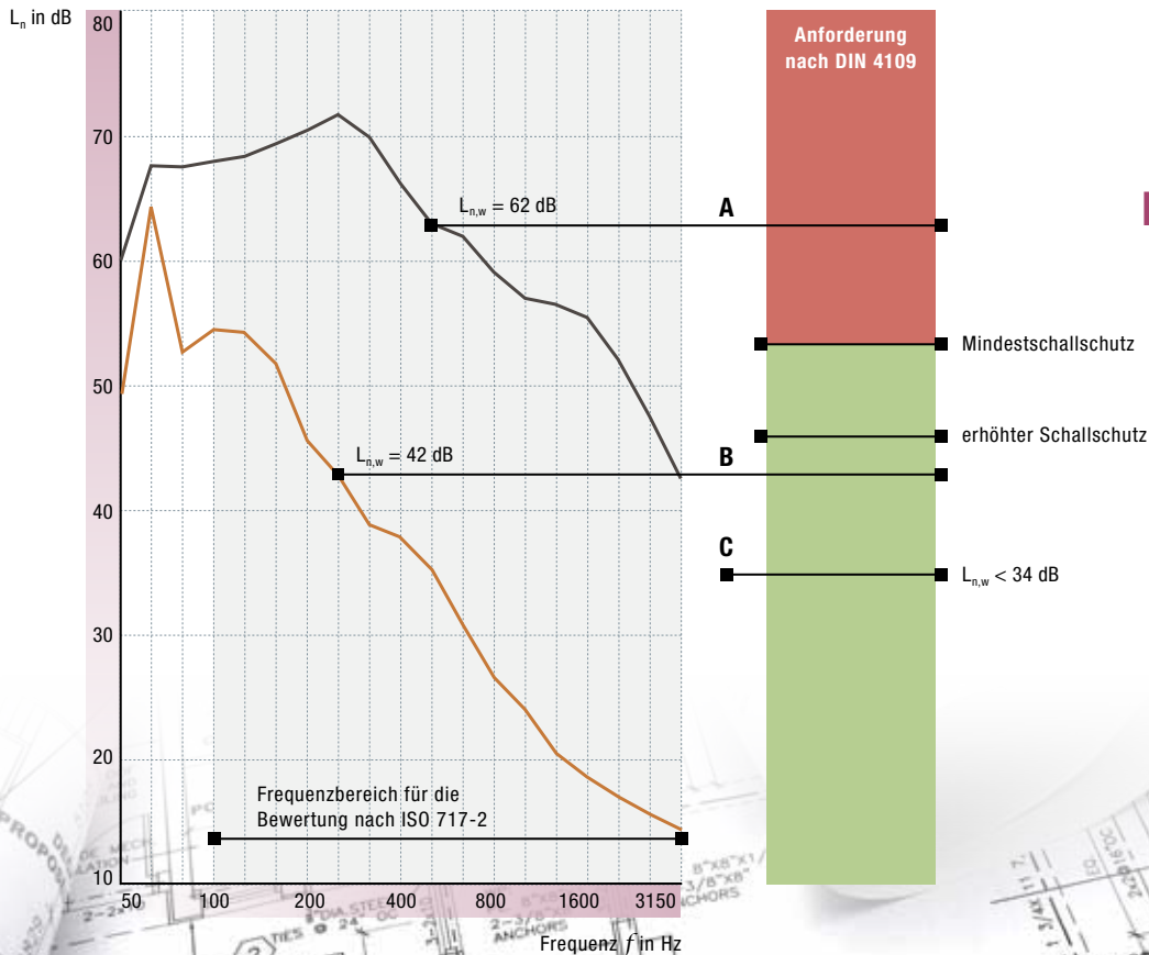
Baustellenmessung
